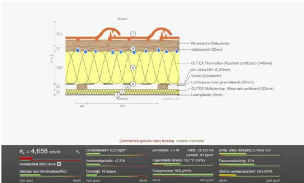
Voorbeeld constructieopbouw uit ubakus inclusief berekening condensatie
